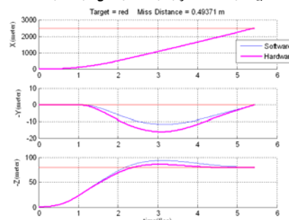
شکل ۱۴- مسیرهای پروازی تک‌بعدی برای سناریوی شماره یک در دو حالت
