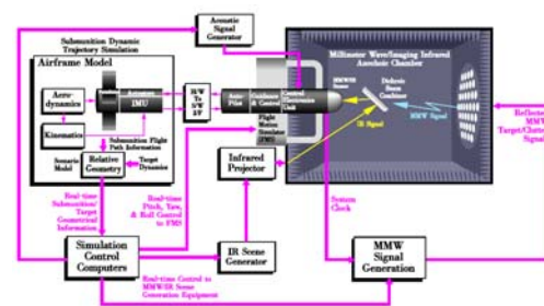
شکل ۱- دیاگرام بلوکی سخت‌افزار در حلقه برای یک موشک مادون قرمز
