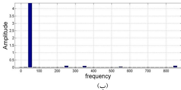
شکل ۵. الف. ولتاژ Back-EMF در حوزه فرکانس، ب. نمای نزدیک
