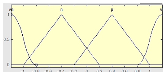
شکل ۶: سیگنال خطا
