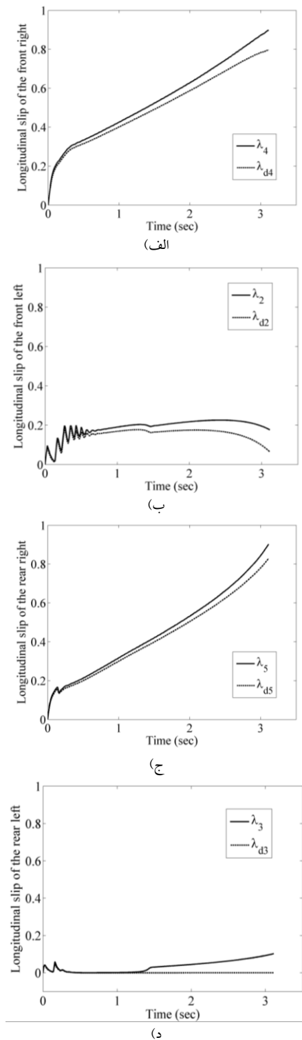
شکل ۸: پاسخ لغزش طولی هر چرخ و مقدار مطلوب آن در سیستم کنترلی پیشنهادی الف) چرخ جلو راست، ب) چرخ جلو چپ، ج) چرخ عقب راست، د) چرخ عقب چپ
