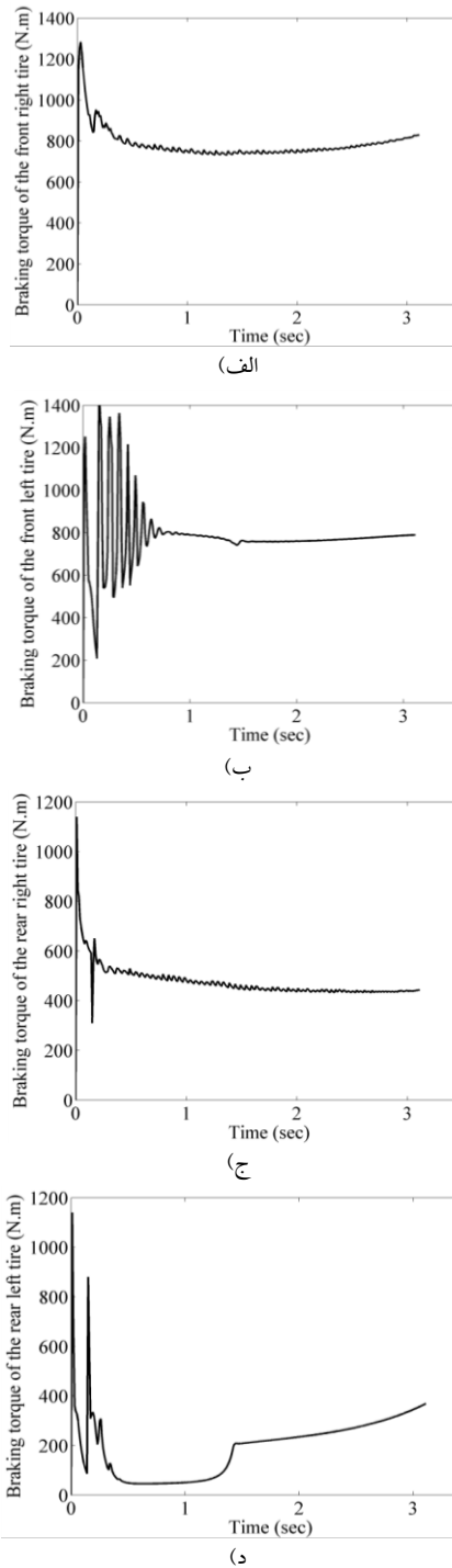
شکل ۷: گشتاور ترمزی هر چرخ در سیستم کنترلی پیشنهادی الف) چرخ جلو راست، ب) چرخ جلو چپ، ج) چرخ عقب راست، د) چرخ عقب چپ
