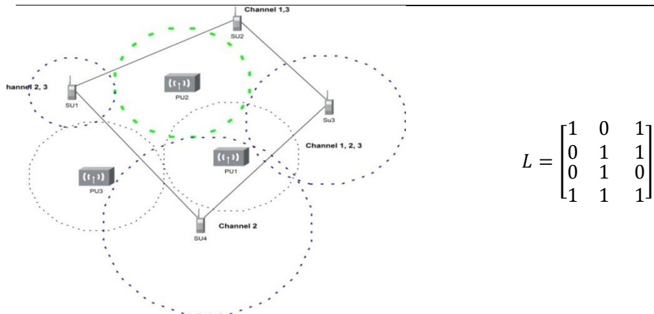
شکل ۱. یک شبکه رادیوی شناختگر با ۳ کاربر اولیه و ۴ کاربر ثانویه ناحیه تحت پوشش این کاربران و ماتریس دسترس‌پذیری آن
