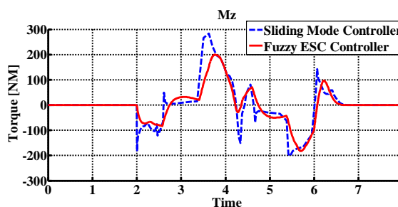
شکل ۲۵: گشتاور اصلاحی خروجی کنترلرها
