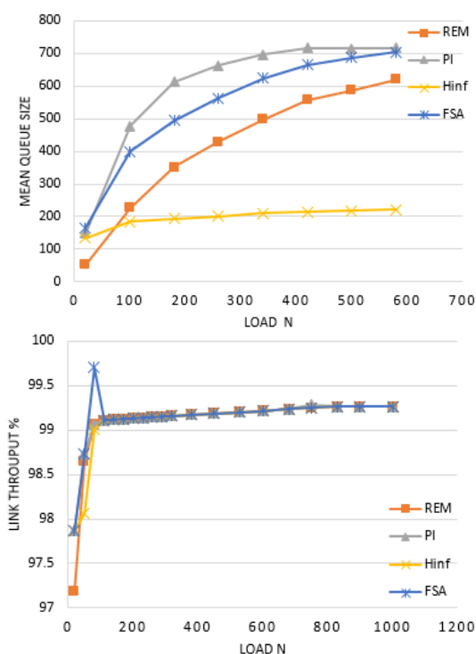
شکل ۱۷: عملکرد کنترل‌کننده‌های مختلف با تغییرات تعداد بار در آزمایش هفتم
