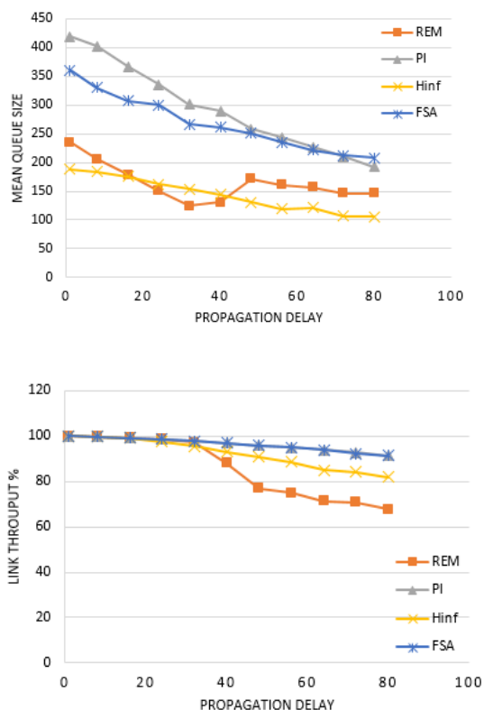
شکل ۱۶: عملکرد کنترل‌کننده‌های مختلف با تغییرات RTT در آزمایش هفتم
