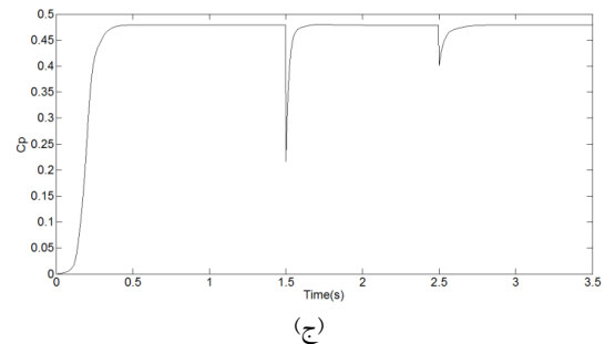
شکل ۱۵: منحنی تغییرات (الف) سرعت باد مرجع (ب) نسبت سرعت نوک (ج) ضریب توان توربین
