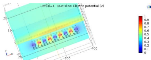
شکل ۳۰: تصویر مربوط توزیع پتانسیل الکتریکی برای تعداد ۴ شانه-نمای ۱
