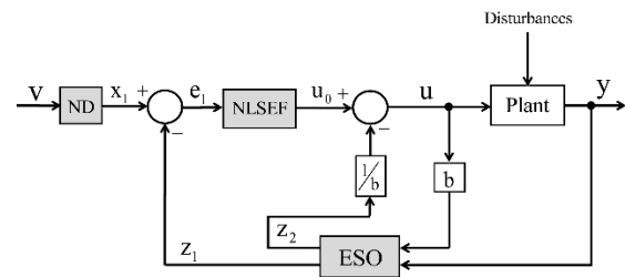
شکل ۲: نمودار روش ADRC
