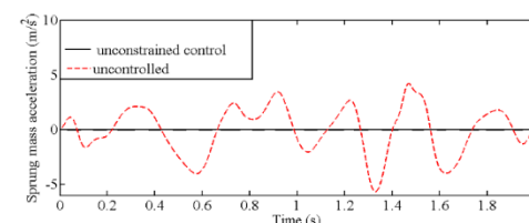
شکل ۱۲: مقایسه‌ی شتاب جرم معلق در سیستم تعلیق فعال نامقید با حالت
