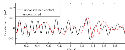
شکل ۱۳: مقایسه‌ی جابه‌جایی تایر در سیستم تعلیق فعال نامقید با حالت
