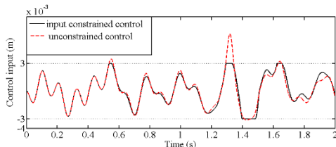
شکل ۱۰: ورودی کنترلی (جابه‌جایی قرقره شیر هیدرولیک) در سیستم تعلیق
