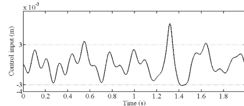
شکل ۱۴: ورودی کنترلی (جابه‌جایی قرقره شیر هیدرولیک) در سیستم تعلیق
