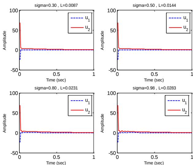
شکل ۲- سیگنال کنترل محاسبه شده توسط کنترل مبتنی بر مدل پیش‌بین و با روش رویداد-تحریک مبتنی بر تابع لیاپانوف با پایداری ورودی به حالت
