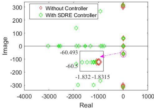
شکل ۵: مقادیر ویژه سیستم در نقطه کار نامی آن (سرعت سنکرون) با حضور کنترل کننده SDRS
