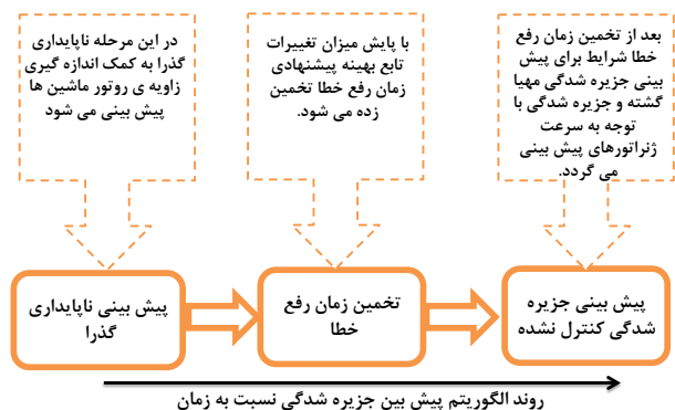
شکل ۲: روند کنترل جزیره شدگی نسبت به زمان
