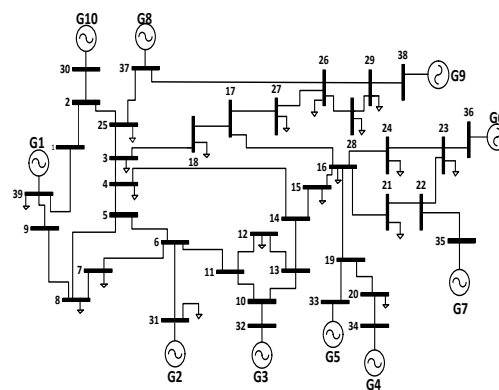
شکل ۵: شبکه ۳۹ باس ۱۰ ماشین استاندارد IEEE
