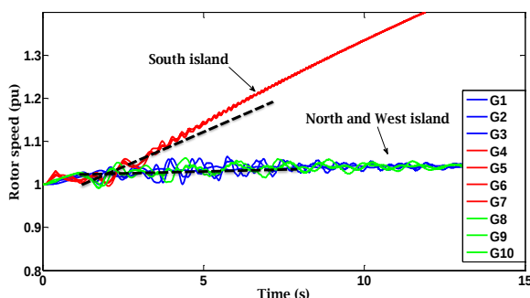
شکل ۱۱: نحوه تغییرات سرعت ژنراتورها بعد از اعمال خطای ۳ فاز در باس ۱۶ و با رفع خطای ۳۰۰ میلی ثانیه
