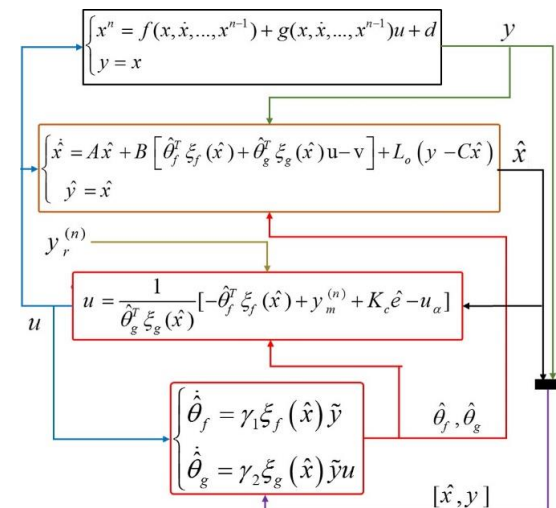
شکل ۲: تصویر مفهومی سیستم کنترل غیر خطی فازی تطبیقی غیر مستقیم همراه با روبتگر فازی تطبیقی
