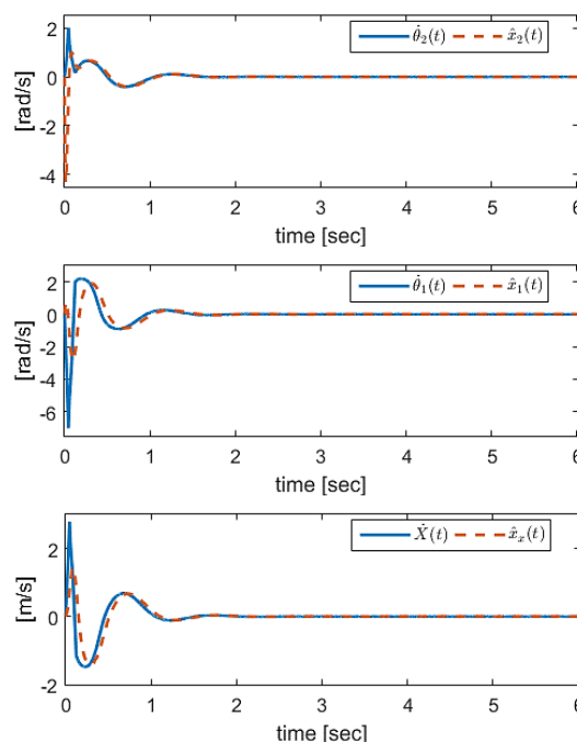
شکل ۵: تغییرات سرعت اجزاء آونگ معکوس دوگانه پس از رها سازی از شرایط اولیه
