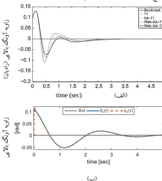
شکل ۱۳: مقایسه نتایج شبیه‌سازی برای زاویه آونگ بالایی. الف) نتایج مقاله با مقایسه روش‌های مختلف ذکر شده در متن مقاله ب) نتایج این پژوهش در شکل ۱۴ مقایسه‌ی بین زاویه آونگ پایینی در هر دو حالت مدل این پژوهش و مرجع اشاره شده، ارائه شده است. تفاوت محرز عملکرد دو رویکرد در شروع فرآیند روشن است.
