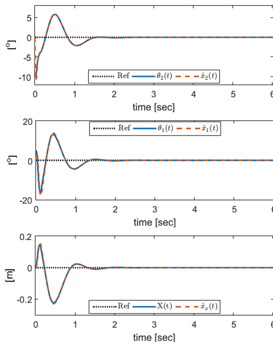
شکل ۴: تغییرات موقعیت اجزاء آونگ معکوس دوگانه پس از رها شدن از شرایط اولیه
