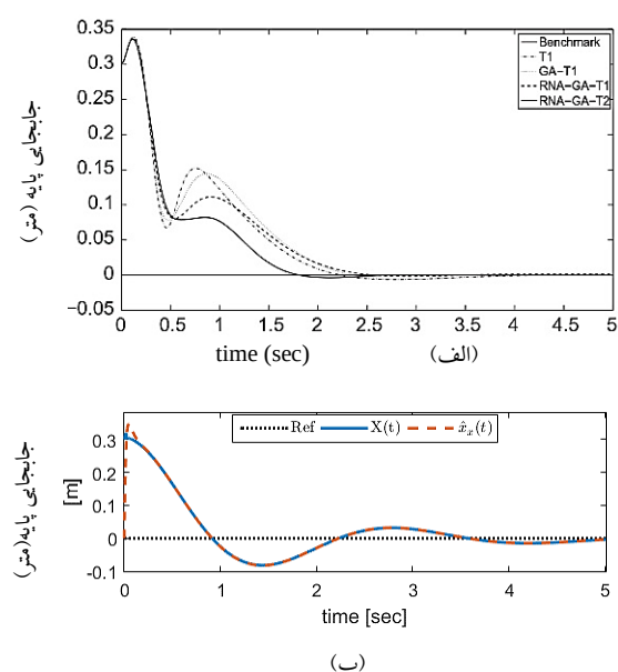
شکل ۱۵: مقایسه نتایج شبیه‌سازی برای جابجایی پایه متحرک. الف) نتایج مقاله با مقایسه روش‌های مختلف ذکر شده در متن مقاله ب) نتایج این پژوهش
