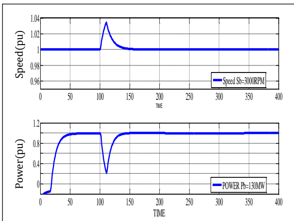
شکل ۱۴: پاسخ مدل توربین گاز به شرایط رده‌بار
