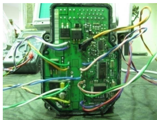
شکل ۱۷: بلوک سیستم ترمز ضد قفل مجهز به سیم های دریافت سیگنال
