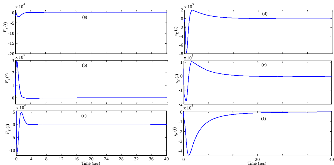
شکل ۸. پاسخ های زمانی ورودی های کنترلی دسته سوم \tau(t) اعمال شده به زیردریایی NPS AUV II. (a): پاسخ زمانی F_X(t) ; (b): پاسخ زمانی F_Y(t) ; (c): پاسخ زمانی F_Z(t) ; (d): پاسخ زمانی \tau_K(t) ; (e): پاسخ زمانی \tau_M(t) ; (f): پاسخ زمانی \tau_N(t) .
