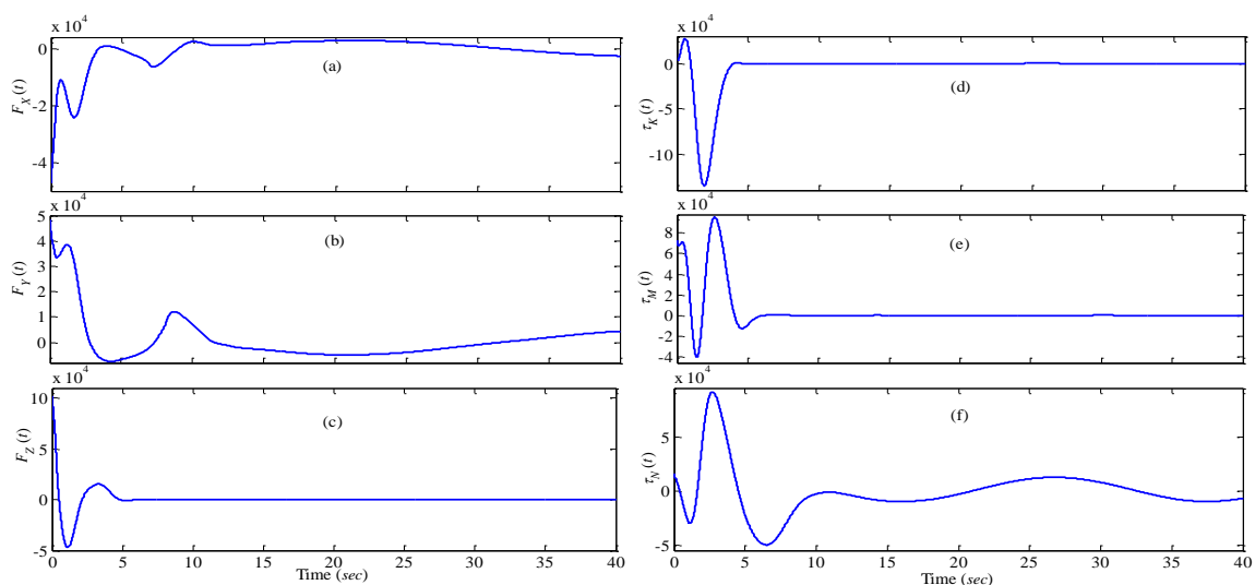
شکل ۶. پاسخ‌های زمانی ورودی‌های کنترلی دسته دوم \tau(t) اعمال شده به زیردریایی NPS AUV II. (a): پاسخ زمانی F_x(t) ; (b): پاسخ زمانی F_y(t) ; (c): پاسخ زمانی F_z(t) ; (d): پاسخ زمانی \tau_x(t) ; (e): پاسخ زمانی \tau_y(t) ; (f): پاسخ زمانی \tau_z(t) .
