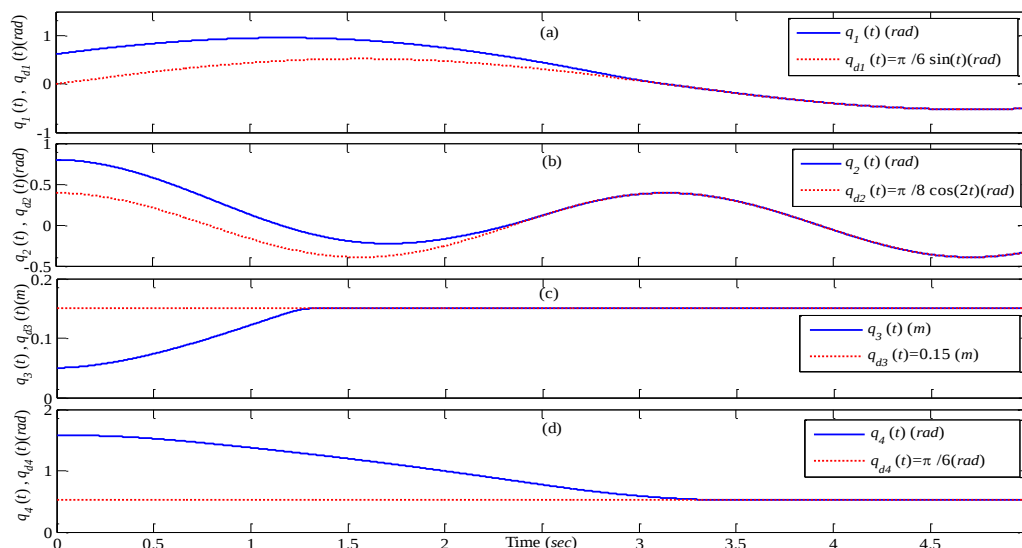
شکل ۱۰. پاسخ‌های زمانی پیگیربندی مفاصل ربات SCARA با اعمال گشتاورهای پیشنهادی دسته چهارم و فرض در نظر گرفتن غیرخطی‌سازهای ناحیه مرده. (a): پاسخ‌های زمانی
