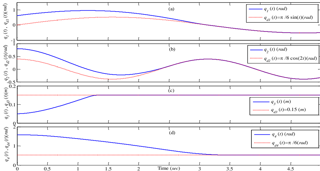
شکل ۱۰. پاسخ‌های زمانی متغیرهای پیکربندی مفاصل ربات SCARA با اعمال گشتاورهای پیشنهادی دسته چهارم و فرض در نظر گرفتن غیرخطی‌سازهای ناحیه مرده. (a): پاسخ‌های زمانی q_1(t) و q_{d1}(t) ; (b): پاسخ‌های زمانی q_2(t) و q_{d2}(t) ; (c): پاسخ‌های زمانی q_3(t) و q_{d3}(t) و q_4(t) و q_{d4}(t) ; (d): پاسخ‌های زمانی q_4(t) و q_{d4}(t)
