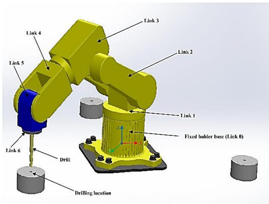
شکل 7. شماتیک مدل شبیه سازی شده ربات IRB-120 توسط نرم افزار solidworks
