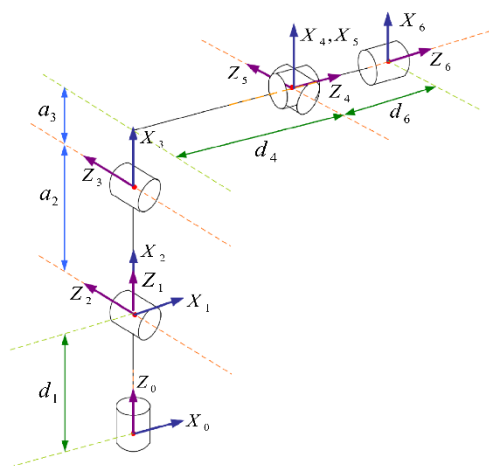
شکل 8. مدل سینماتیکی ساده شده ربات IRB-120
