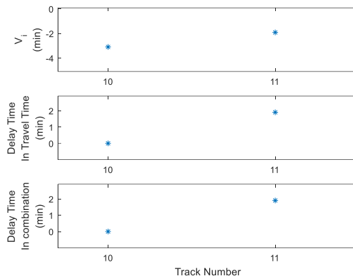
شکل ۱۰: نمایش متغیر کنترلی V_i ، تأخیر زمانی در حالت کنترل با روش کاهش زمان سفر و کنترلی ترکیبی
