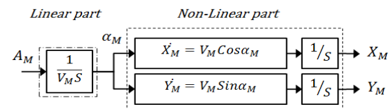
شکل (۳) تفکیک اجزاء سینماتیک حرکت موشک به دو بخش خطی و غیرخطی
