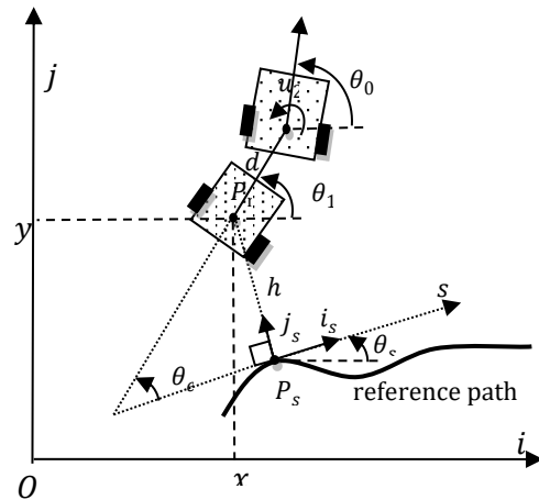
شکل ۱: ربات متحرک دارای تریلر و مسیر مرجع
