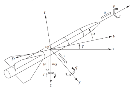
شکل ۲- نیروهای وارد شده بر موشک [۳۶]
