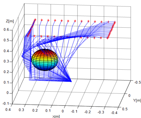
شکل ۸: پیکربندی‌های نهایی ربات در حالت نامعید
