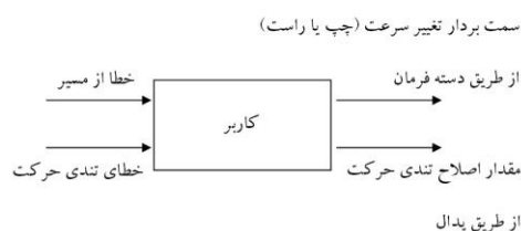
شکل ۱. نمودار ورودی ها و خروجی های الگوریتم هدایت
