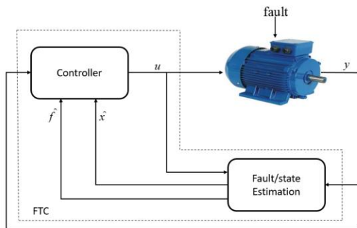
شکل ۱: ساختار کلی سیستم کنترل کننده تحمل پذیر عیب مبتنی بر تخمین عیب
