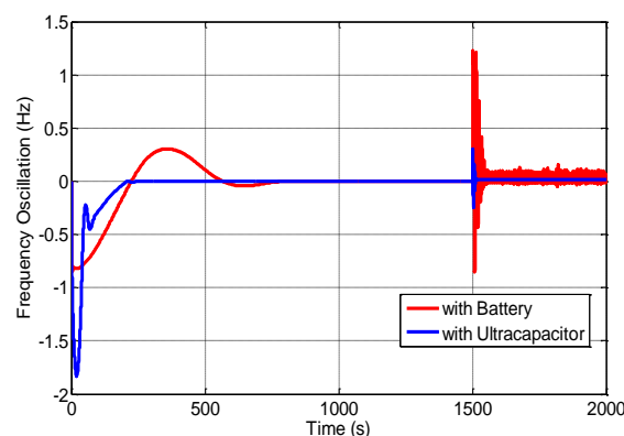
شکل ۱۳: مقایسه رفتار فرکانسی ریزشبهه در حضور باتری و ابرخازن
