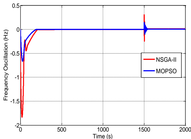
شکل ۱۵: مقایسه رفتار فرکانسی ریزشبهه با اعمال الگوریتم‌های بهینه
