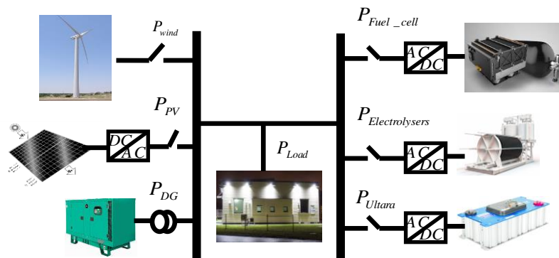
شکل ۱: دیاگرام تک خطی ریزشیکه مورد مطالعه با اعمال تاخیر سیستم مخابراتی
