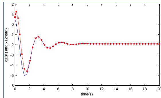
ج- نمایش دومین متغیر حالت زیر سیستم اول به همراه تخمین آن شکل ۱- رویکر غیر متمرکز با ورودی نامعین برای زیر سیستم اول (خط توپر: متغیر حالت و خط-نقطه: تخمین متغیر حالت)
