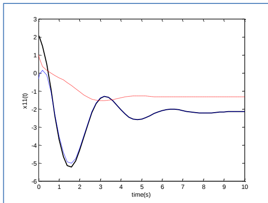
الف- نمایش اولین متغیر حالت زیر سیستم اول با استفاده از روش پیشنهادی و رویکر لیونبرگر
