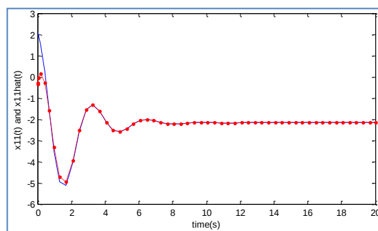
ب- نمایش اولین متغیر حالت زیر سیستم اول به همراه تخمین آن توسط روینگر از مرتبه ۲ با ورودی نامعین
