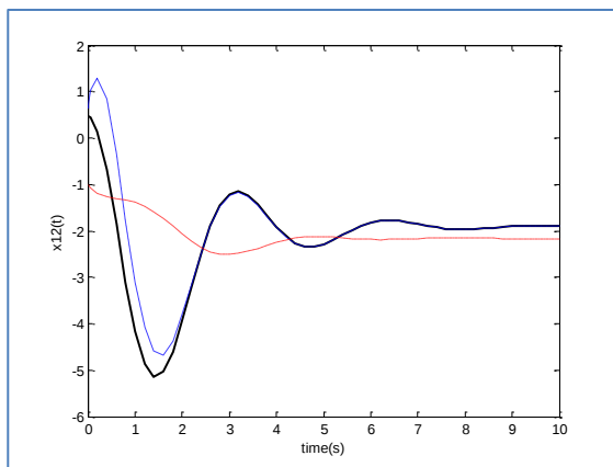
ب- نمایش دومین متغیر حالت زیر سیستم اول با استفاده از روش پیشنهادی و رویکر لیونبرگر
