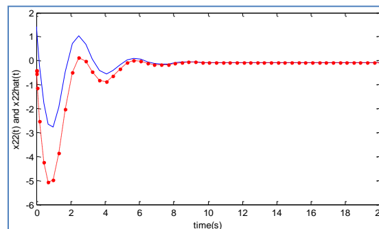
ج- نمایش دومین متغیر حالت زیر سیستم دوم به همراه تخمین آن شکل ۲- روینگر غیر متمرکز با ورودی نامعین برای زیر سیستم دوم (خط توپر: متغیر حالت و خط-نقطه: تخمین متغیر حالت)
