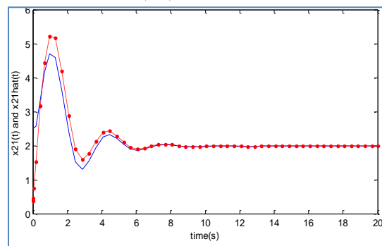
ب- نمایش اولین متغیر حالت زیر سیستم دوم به همراه تخمین آن توسط روینگر از مرتبه ۲ با ورودی نامعین
