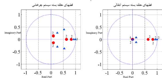
شکل ۷: قطب‌های حلقه بسته سیستم‌های انتقالی و چرخشی هگزاروتور
