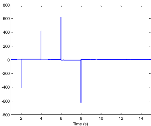
شکل ۴: مانده طراحی شده به کمک روش پربیتی غیرخطی
