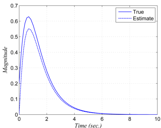
شکل ۳: منحنی های x_2(t) و \hat{x}_2(t) برای سامانه حلقه-بسته بدون اغتشاش
