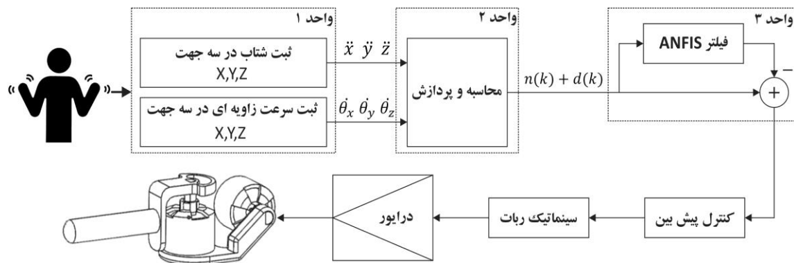
شکل ۲: طرح کلی سیستم پیشنهادی
