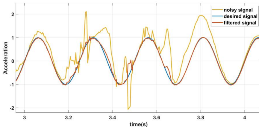
شکل ۶: مقایسه سیگنال حاصل از فیلتر ANFIS و سیگنال دارای نویز
