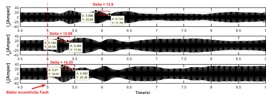
شکل ۹- جریان های موتور القایی در شرایط عیب سناریوی اول
