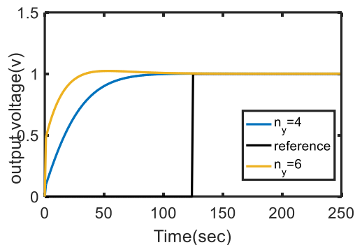
شکل ۱۰. مقایسه خروجی مبدل باک در دو افق پیش بین n_y = 4, 6 .
