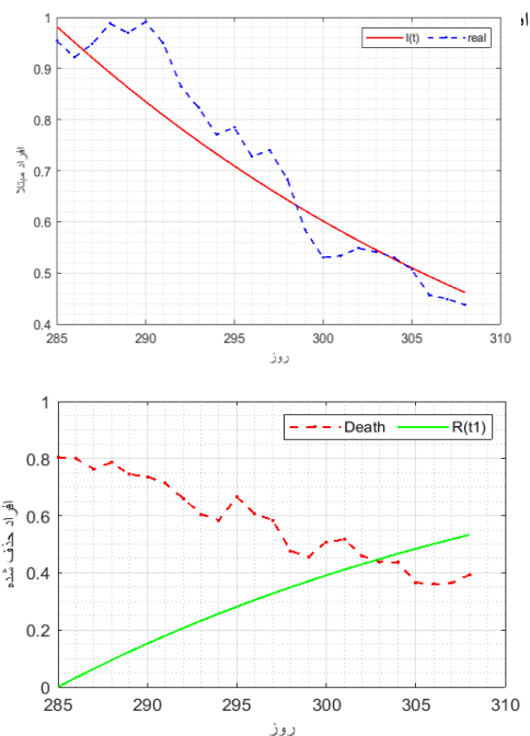
شکل ۶. الف) نمودار مقایسه افراد مبتلا شده در بازه پنجم و تخمین مدل از افراد مبتلا ( a = 0/73 و b = 0/33 ). ب) نقاط قرمز رنگ تعداد افراد فوت شده در اثر کرونا و خط سبز رنگ تخمین مدل از افراد حذف شده در بازه پنجم.
