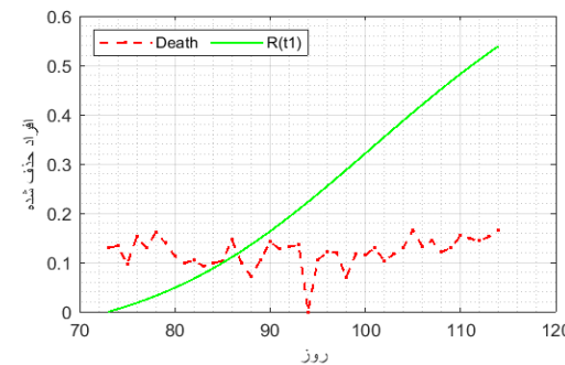
شکل ۳. الف) نمودار مقایسه افراد مبتلا شده در بازه دوم و تخمین مدل از افراد مبتلا (a = 0/17 و b = 0/082) . ب) نقاط قرمز رنگ تعداد افراد فوت‌شده در اثر کرونا و خط سبز رنگ تخمین مدل از افراد حذف‌شده در بازه دوم.
