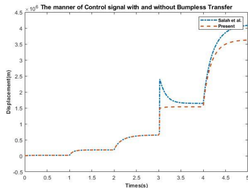
شکل ۱۱: مقایسه رفتار سیگنال کنترل در زمان کلیدزنی برای مدل‌های برگزیده تکه‌ای حاضر
