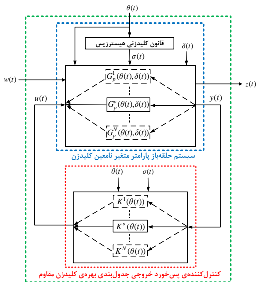
شکل ۲: سیستم حلقه‌بسته‌ی پارامتر متغیر خطی نامعین کلیدزن
