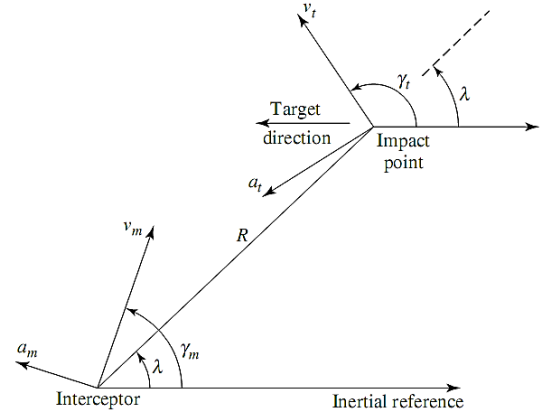
شکل ۳: هندسه دو بعدی درگیری موشک و هدف [۱۴]
