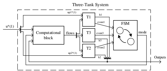
شکل ۵: شماتیک مدل‌سازی سیستم سه مخزن در سیمولینک
