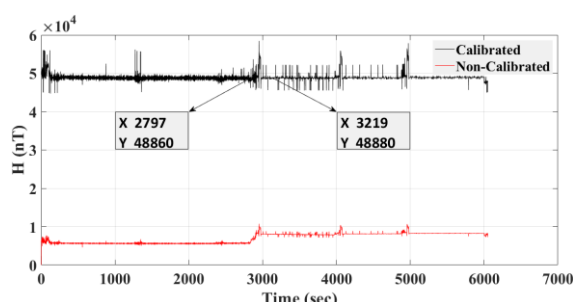
شکل 12: اندازه‌ی میدان مغناطیسی در آزمون دوم بعد از اصلاح نهایی ضرایب کالیبراسیون
