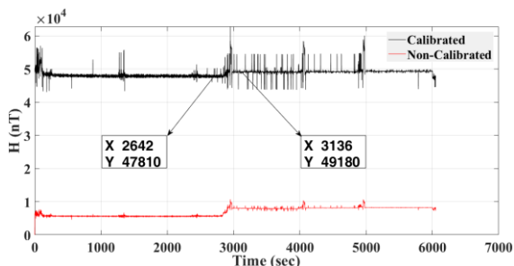
شکل ۸: اندازه‌ی میدان مغناطیسی در آزمون دوم قبل و بعد از اعمال ضرایب
