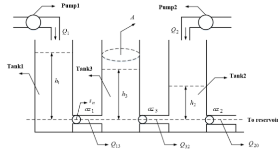
شکل ۲. شماتیک سیستم سه تانک [۱]
