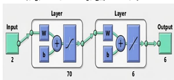
شکل ۱: ساختار شبکه عصبی
