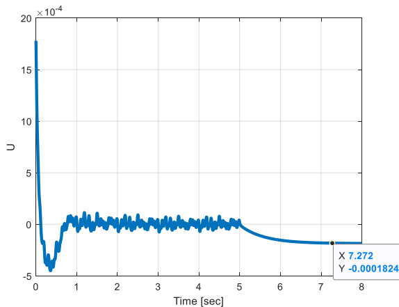
شکل ۵: سیگنال کنترلی
