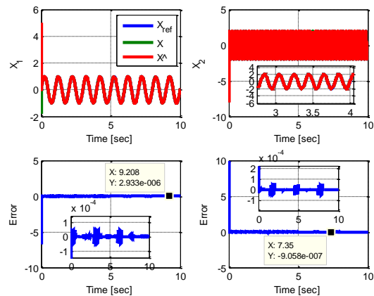
شکل ۱۱: مسیر مرجع، متغیرهای حالت سیستم اصلی، رویکرد و خطای بین آنها
