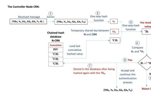
شکل ۱: ایجاد زنجیره چکیده جمعی در گره حسگر و کنترل‌کننده [۲۱]
