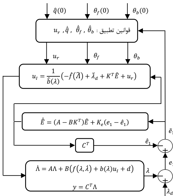
شکل ۴: ساختار پیاده‌سازی کنترل‌کننده فازی تطبیقی غیرمستقیم مقاوم بر اساس رویکنگر برای سیستم ترمز ضد قفل
